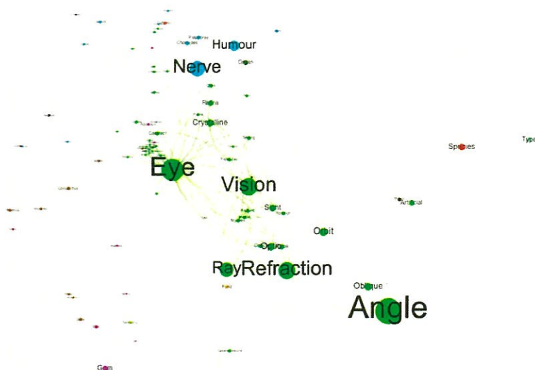
Fig. 6. 'Eye'
